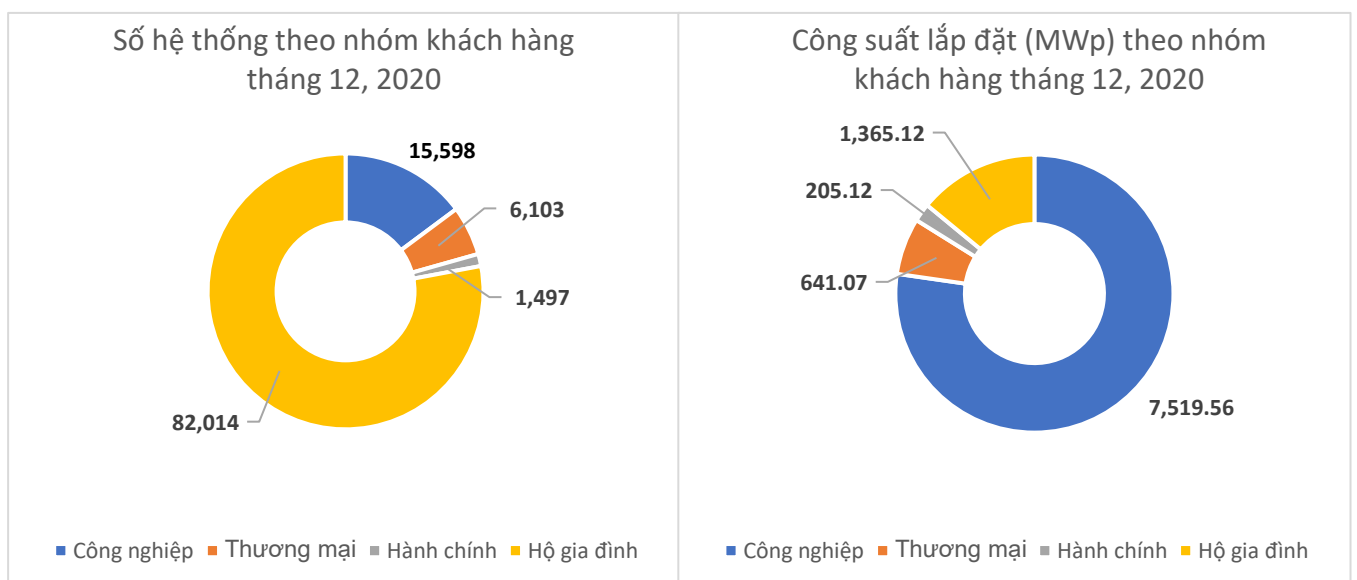
Hình 8. Phân chia hệ thống và công suất ĐMT áp mái theo nhóm khách hàng - tháng 12, 2020
