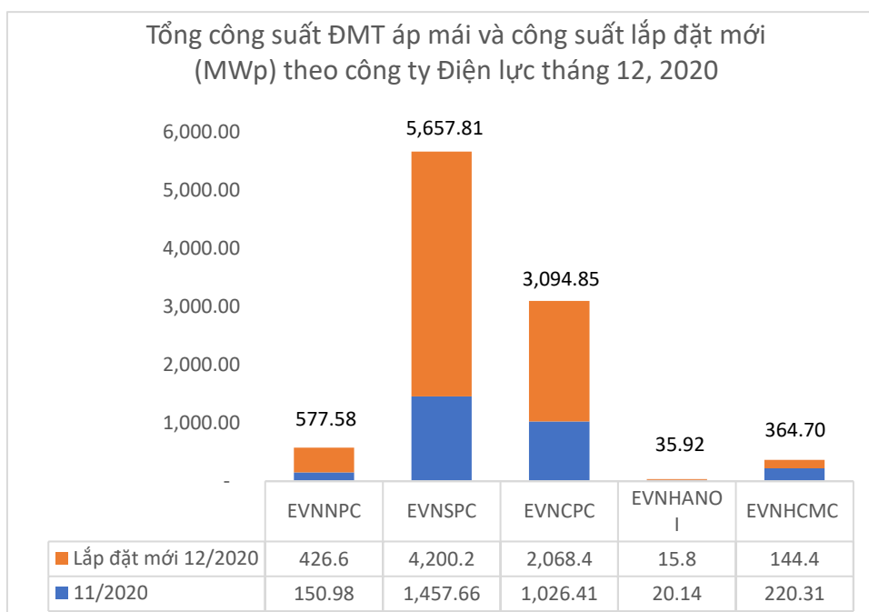
Hình 4. Tổng công suất ĐMT áp mái và công suất lắp đặt mới (MWp) theo công ty Điện lực trong tháng 12, 2020
