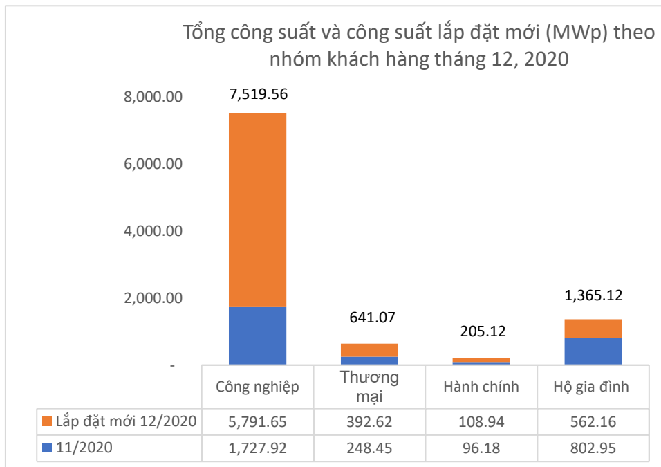
Hình 7. Tổng số công suất lắp đặt và công suất lắp đặt mới (MWp) theo nhóm khách hàng trong tháng 12, 2020
